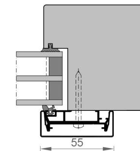
Festverglasung
