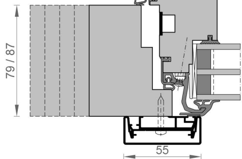
Integralfenster
