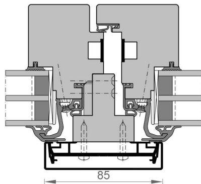
Stulpfenster
