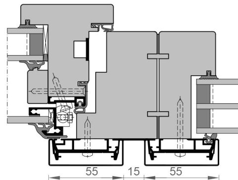
Verbundfenster - Elementkopplung
